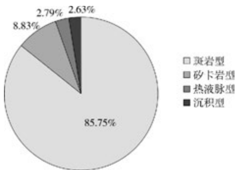
图 1 中国钼矿床成矿类型所占的资源比例 (数据来源:[1])
