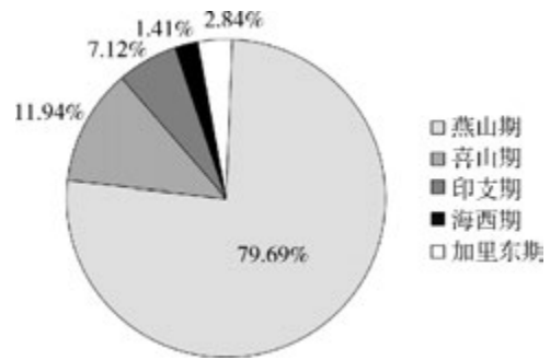
图2 中国钼矿床成矿时代所占的资源比例
